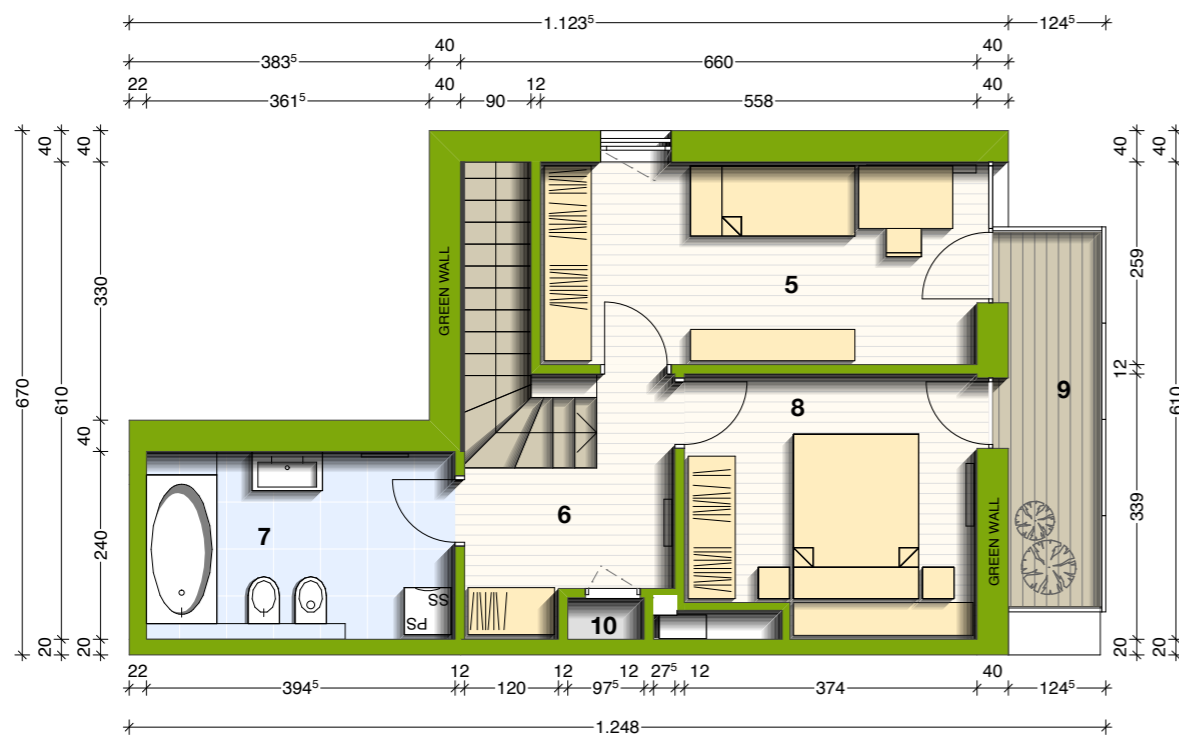
stanovanje - tloris 11. etaže
