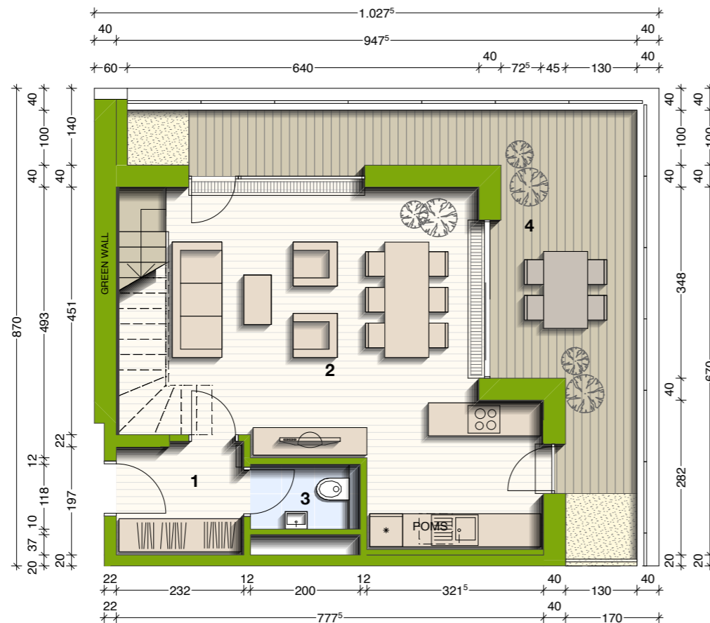
stanovanje - tloris 10. etaže
