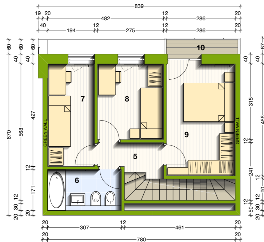
stanovanje - tloris 10. etaže
