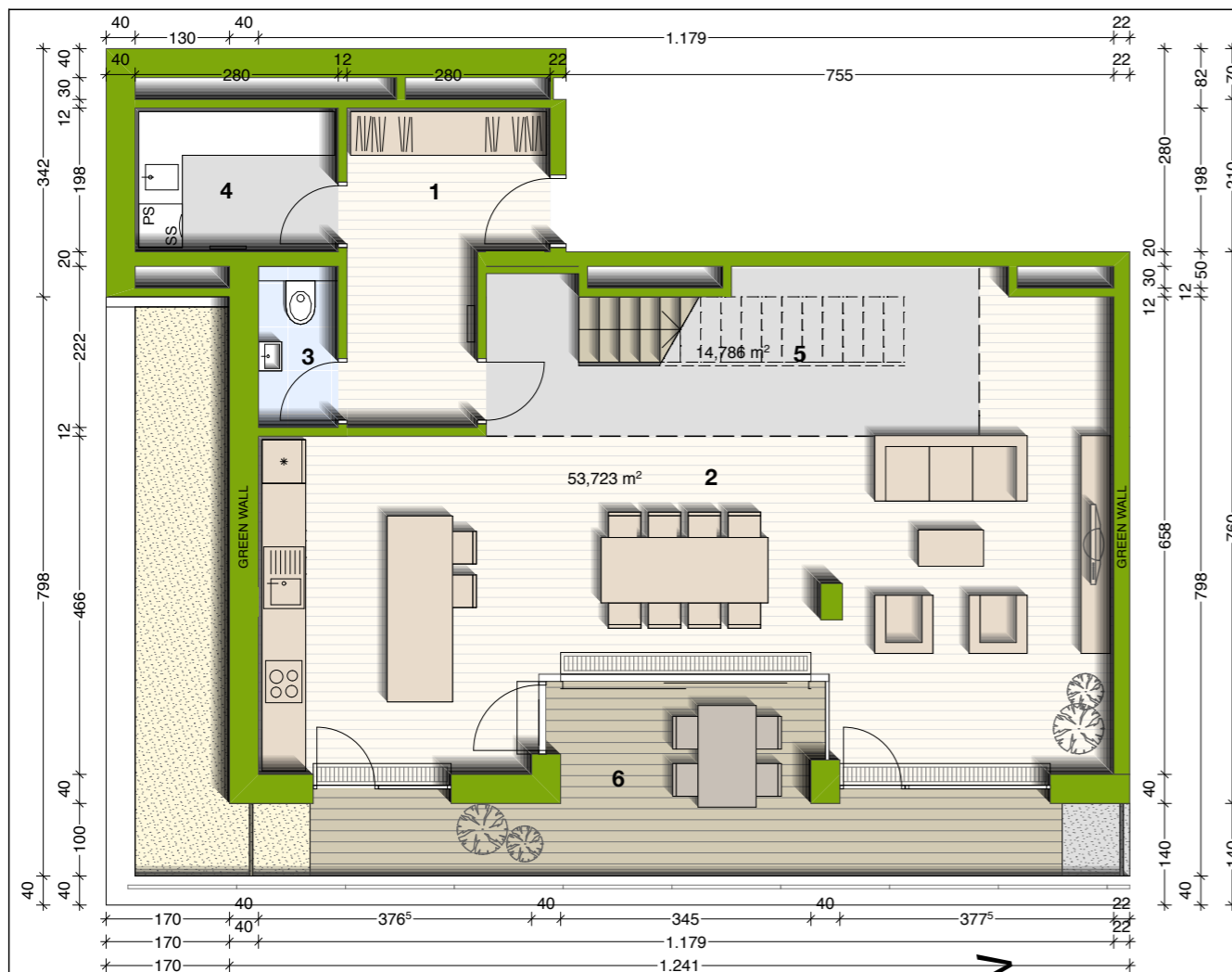
stanovanje - tloris 10. etaže
