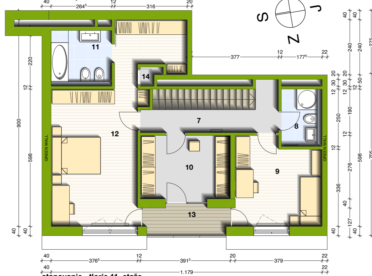
stanovanje - tloris 11. etaže
